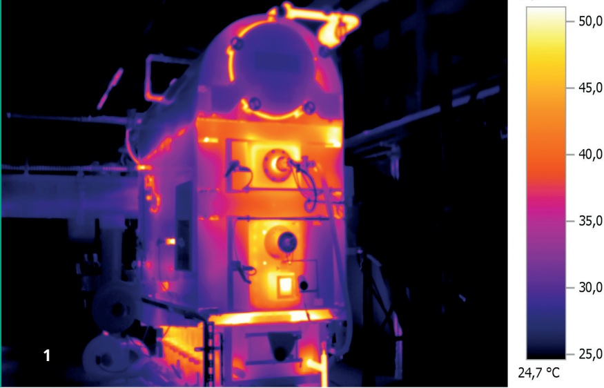
1 Wärmebild unseres Brennofens.
